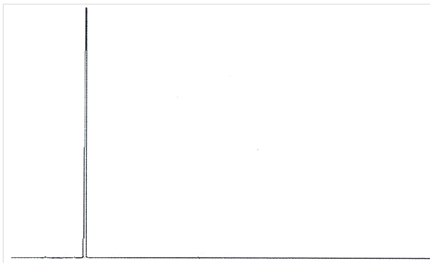
图 B.1 食品添加剂二烯丙基硫醚气相色谱图
